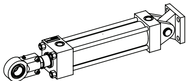
CK-安装形式C, 带附件C-144和C-136
