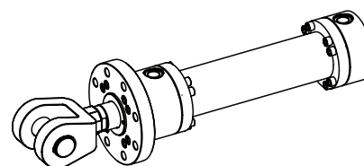
CC-安装形式A, 带附件C-141
