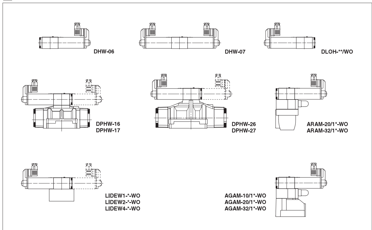
22 本质安全阀的外观示意图
