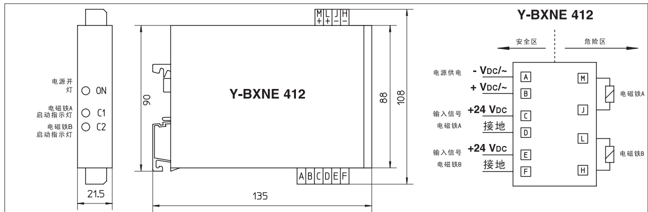
21 安装尺寸[mm]
