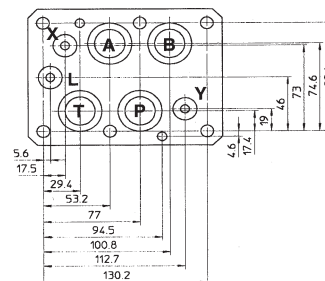
X向视图
