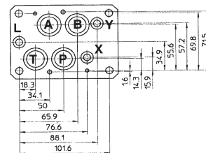
X向视图
