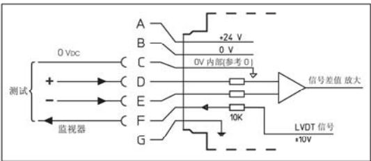
图B 误差信号不接地（浮动连接）
