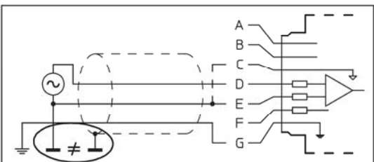
图H 有电位差是时不要将屏蔽线与地面设备连接
