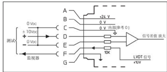
图A 电源和信号共零
