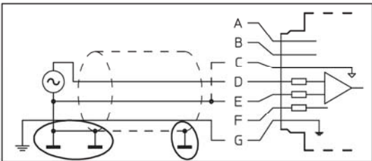
图G 不要将屏蔽线两边都接地
