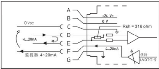
图D 误差输入信号
