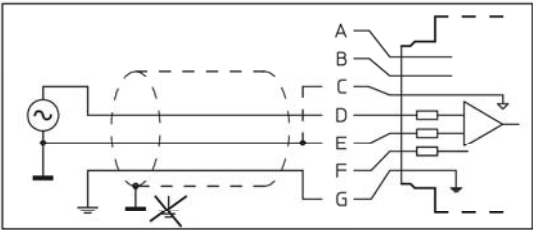
图F 屏蔽线接电源地线GND
