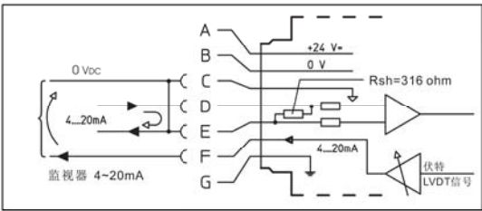
图C 共零
