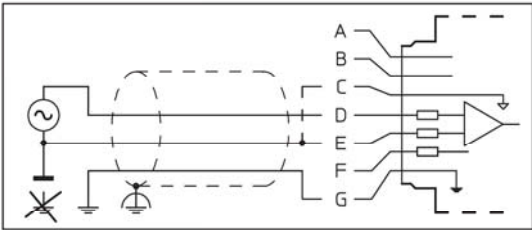
图E 屏蔽线接地保护
