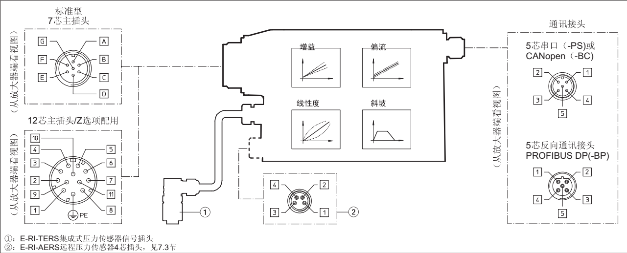
7.1 7芯&12芯插头的电气连接
