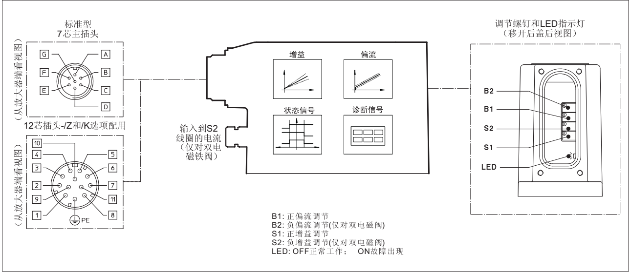
8.1 -TE型阀的电气连接-7芯和12芯接头
