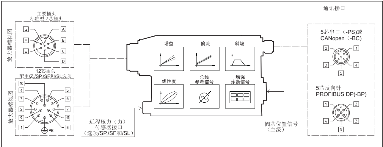
10.1 -LES型阀的电气连接-7芯&12芯接头
