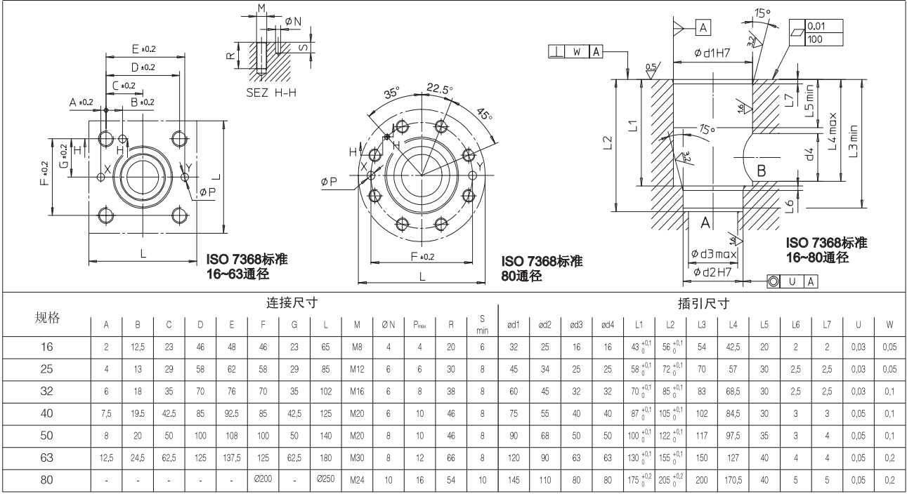
14 盖板连接尺寸和插件腔尺寸[mm]
