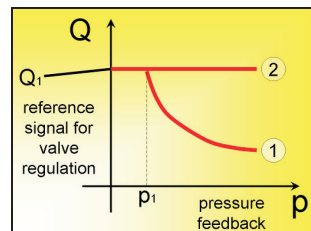
E-BM型调节曲线：①带功率限制曲线，②不带功率限制 p_1 \times Q_1 = 最大功率限制
