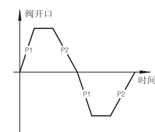
/RR选项-上下不对称斜坡
