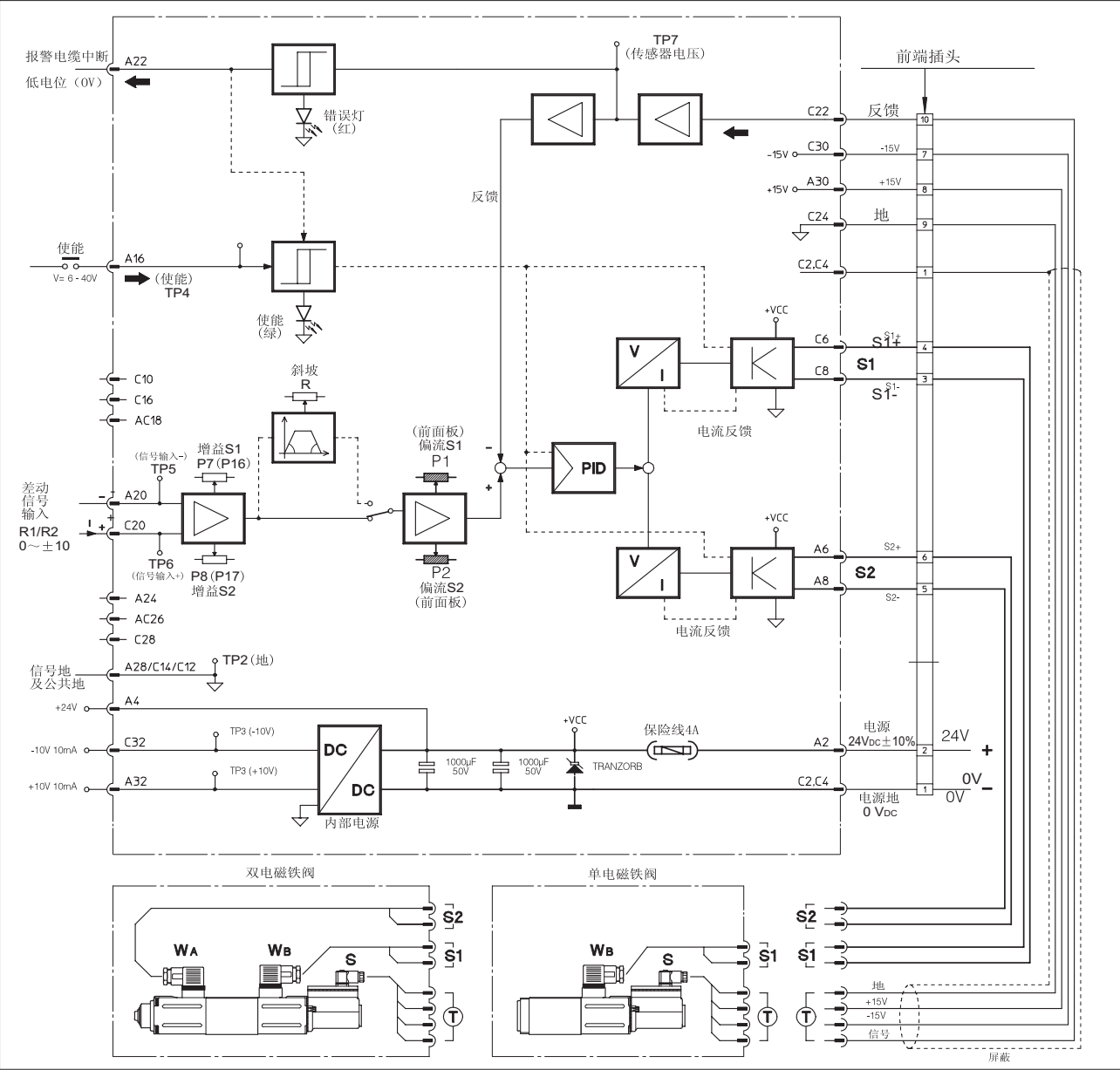
10 接线方框图 (对每个放大器)
