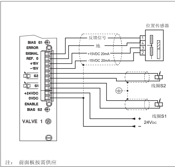
12 前面板接线图 (对每个放大器)
