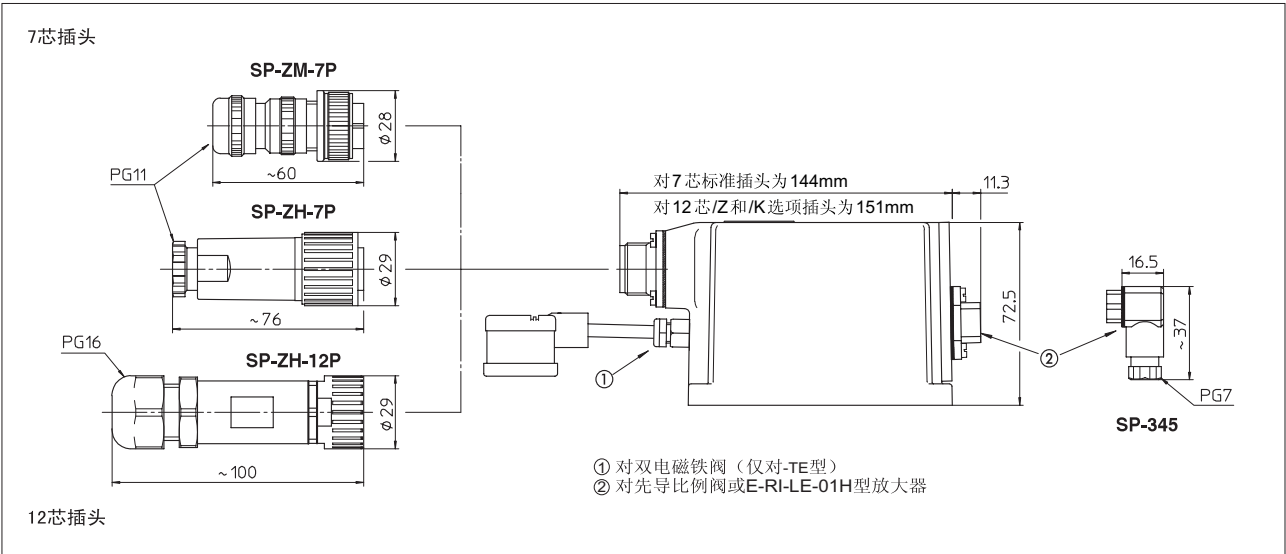
10 电子放大器及插头尺寸 [mm]
