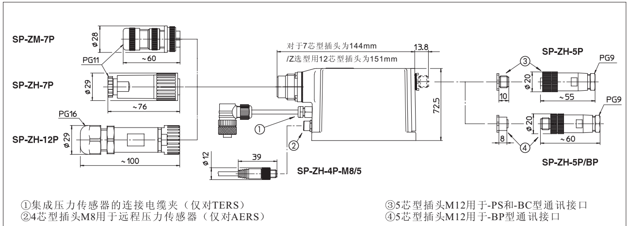
14 外形尺寸[mm]
