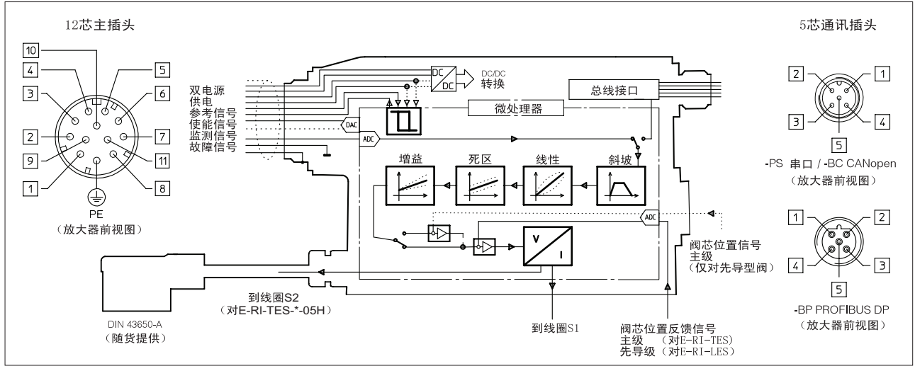
4 7 芯和 12 芯主插头的电气联接
