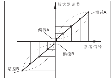
12.7 - 线性度
