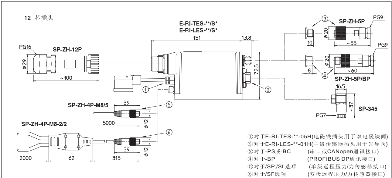
17 外形尺寸[mm]
