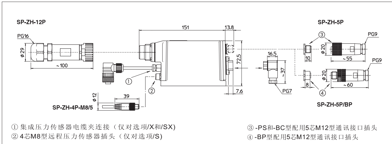
15 外形尺寸[mm]
