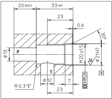
12 SP-CART M-5/**的安装尺寸
