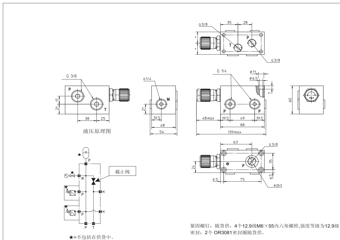
14 BA-244/0/SA型底板的外型尺寸
