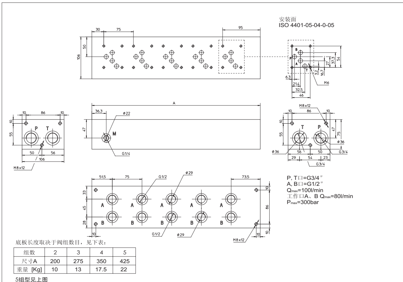
8 BA-314/* /P底板的外形尺寸 (mm)
