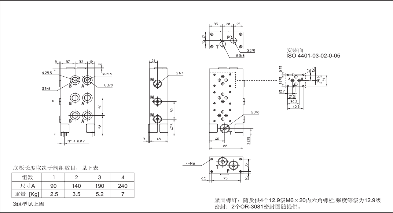
10 BA-244/M5底板的外型尺寸 (mm)
