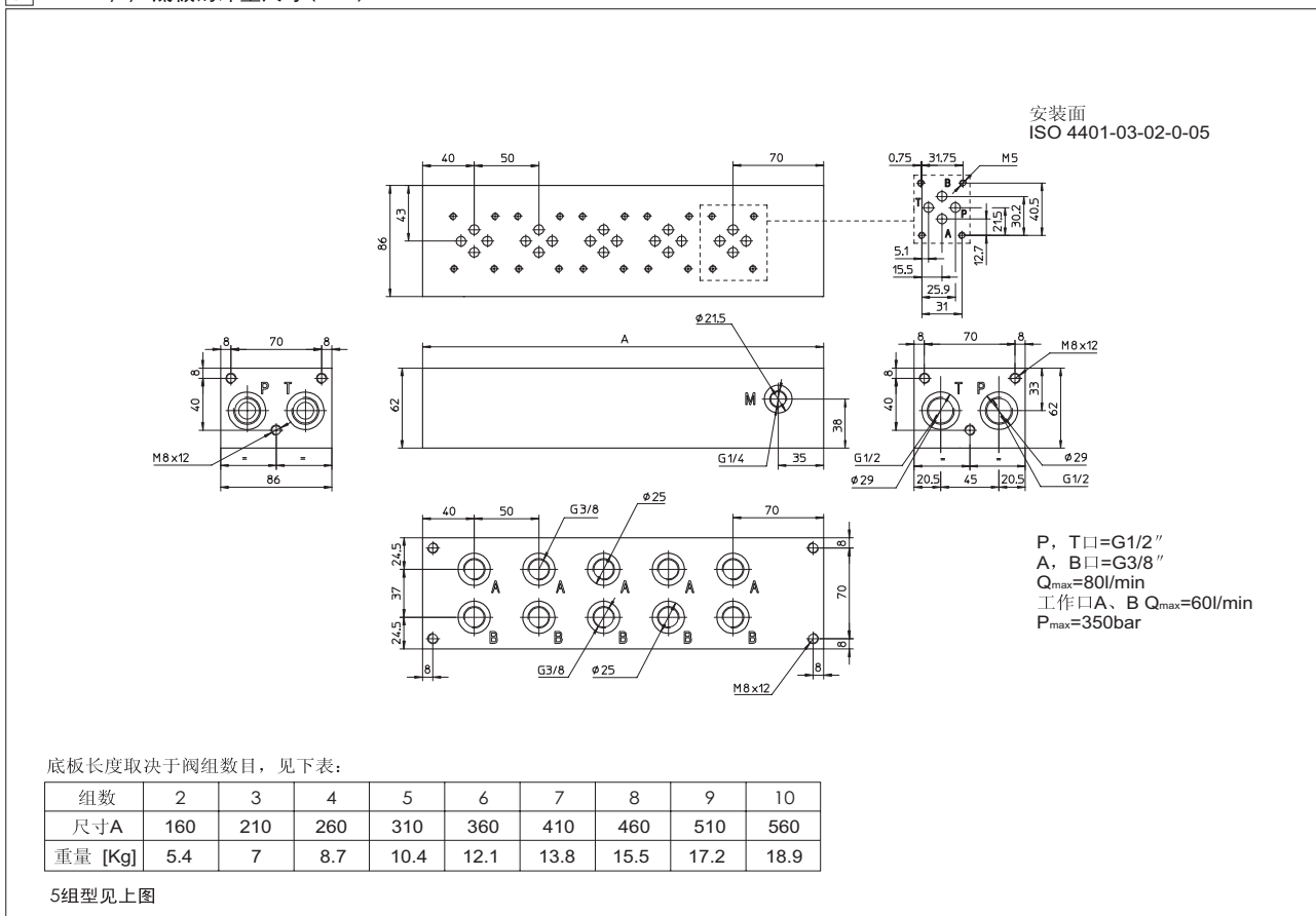
7 BA-214/* /P底板的外形尺寸 (mm)
