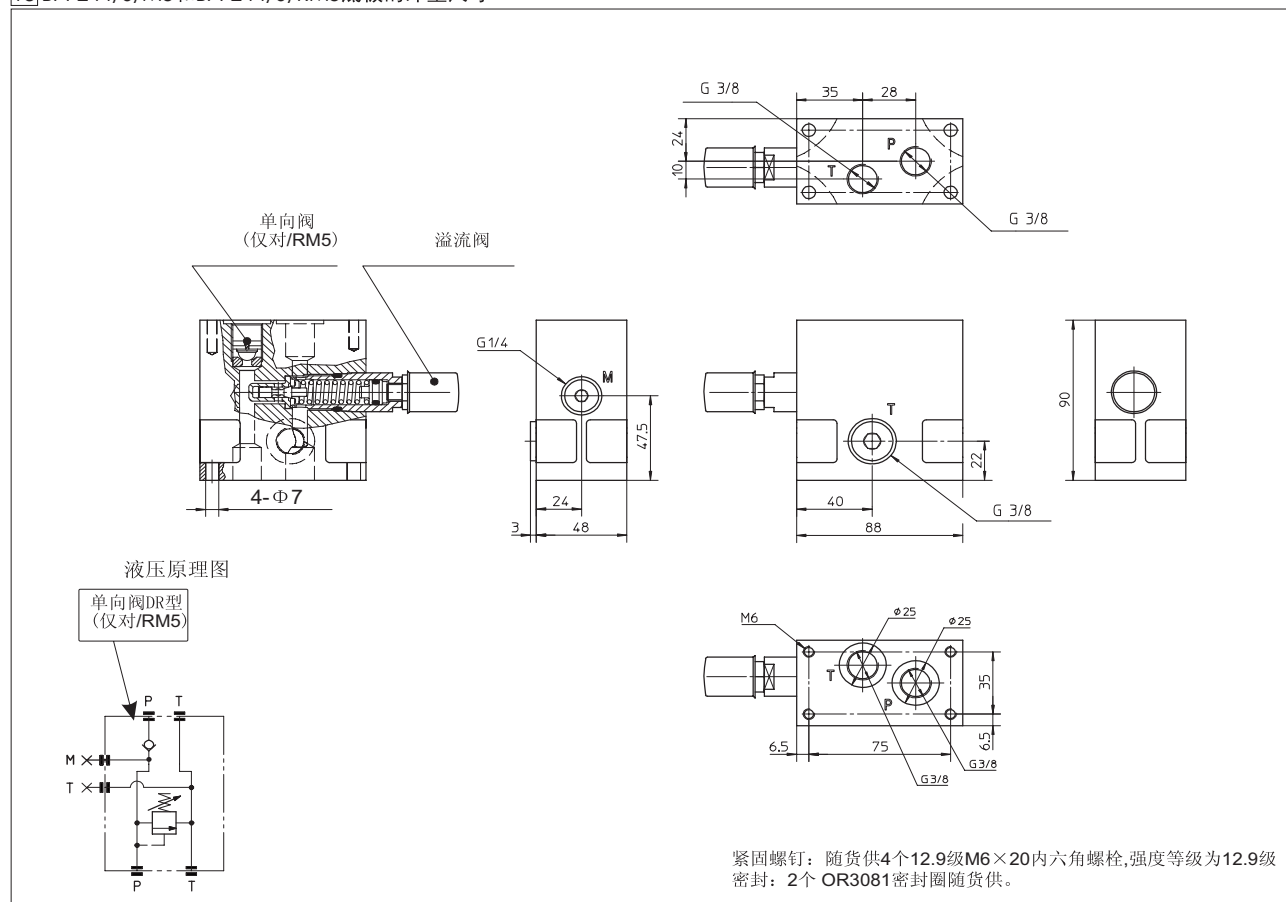
13 BA-244/0/M5和BA-244/0/RM5底板的外型尺寸
